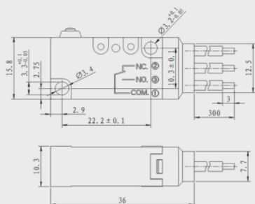
·枢轴短手柄型 XV-101-CW
