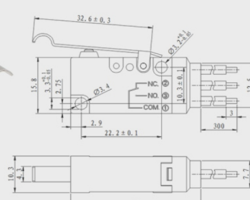
·枢轴滚筒短手柄型 XV-105-CW
