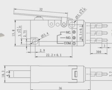
·枢轴长手柄型 XV-103-CW
