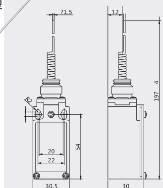
• 万向式触须端头弹簧摇杆型 XZ-9106M
