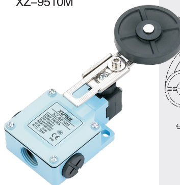
• 可调大滚轮摆杆型 XZ-9510M
