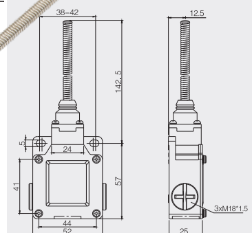
• 万向式金属端头弹簧摇杆型 XZ-9509M
