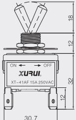
• 四极单向自动复位型 FPST Auto Reset (ON)-OFF XT-41AF
