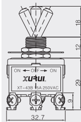
• 四极双投中间停型 FPDT ON-OFF-ON XT-43B
