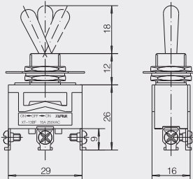
• 单极双向自动复位型 SPDT Auto Reset(ON)-OFF-(ON) XT-13BF
