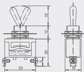
• 单极单向自动复位型 SPST Auto Reset (ON)-OFF XT-11BF
