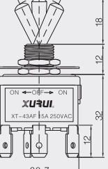
• 四极双向自动复位型 FPDT Auto Reset (ON)-OFF-(ON) XT-43AF
