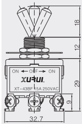
• 四极双向自动复位型 FPDT Auto Reset (ON)-OFF-(ON) XT-43BF
