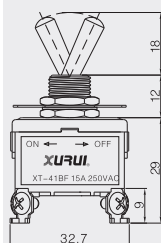
• 四极单向自动复位型 FPST Auto Reset (ON)-OFF XT-41BF
